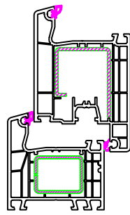
140x07 & 140x30 Frame & Sash • Inward opening door
